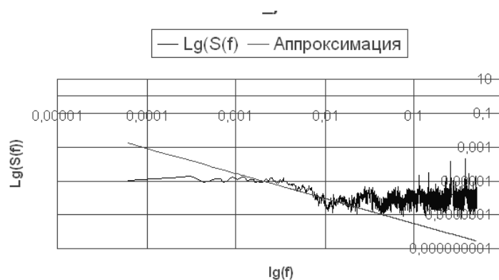
Рисунок 16 - Спектральная плотность временного ряда UDP_j512
