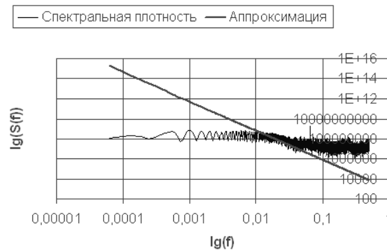
Рисунок 13 - Спектральная плотность временного ряда UDP_d64
