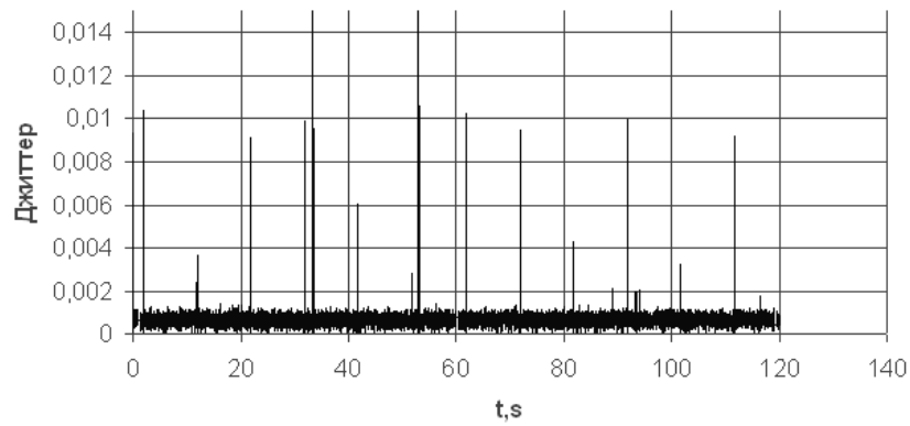
Рисунок 2- Джиттер при передаче пакетов об'ємом 64 байт
