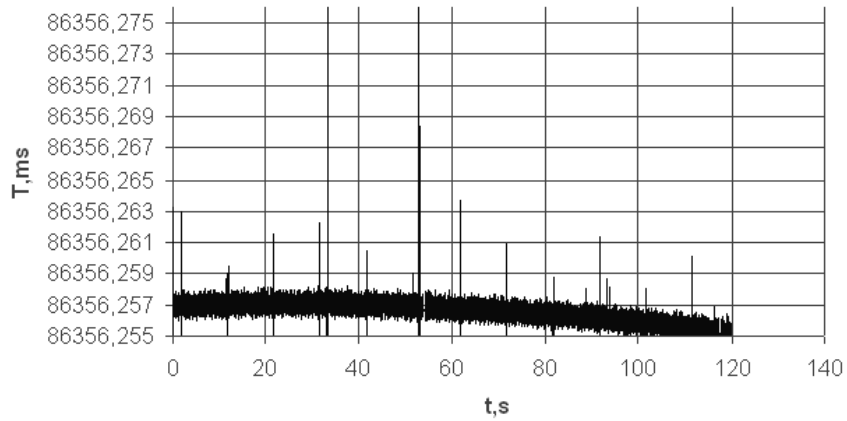
Рисунок 1- Задержка при передаче пакетов об'ємом 64 байт
