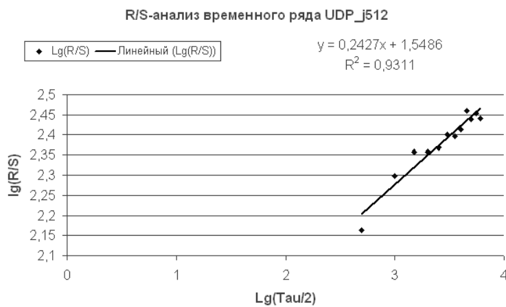
Рисунок 20 - Результат R/S-анализа временного ряда UDP_j512
