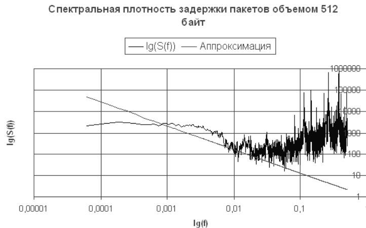
Рисунок 15 - Спектральная плотность временного ряда UDP_d512
