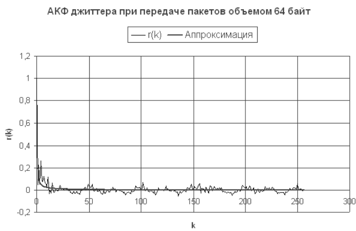
Рисунок 10 - АКФ временного ряда UDP_j64
