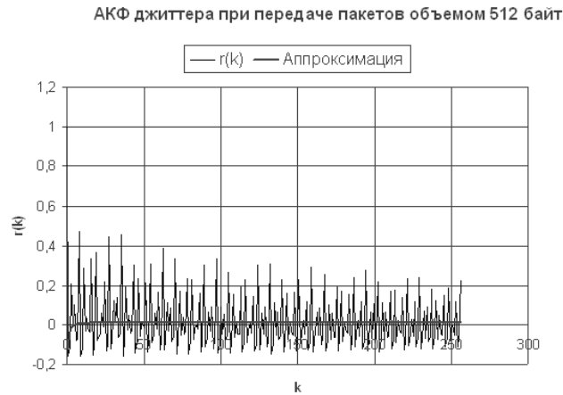
Рисунок 12 - АКФ временного ряда UDP_j512
