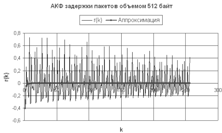
Рисунок 11 - АКФ временного ряда UDP_d512
