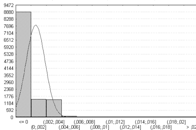
Рисунок 8 - Плотность распределения временного ряда UDP_j512
