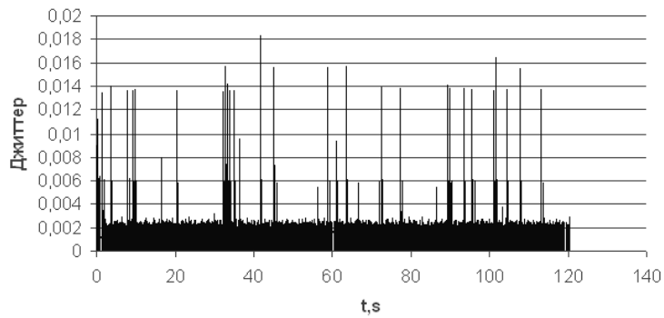
Рисунок 4- Джиттер при передачі пакетов об'ємом 512 байт
